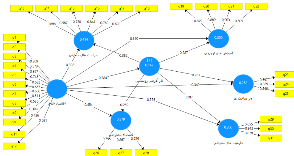
شکل ۳. ضرایب مسیر
