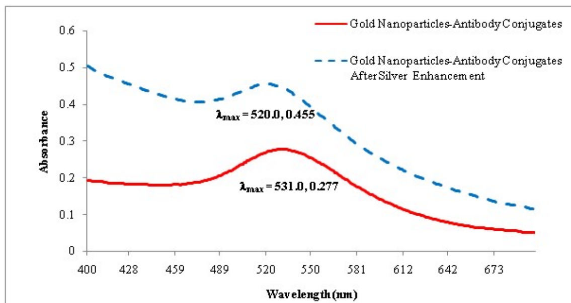
شکل ۵- طیف LSPR تأیید کننده تقویت نقره کانجوه‌های نانوذرات طلا-آنتی بادی؛ طیف LSPR کانجوه‌های نانوذرات طلا-آنتی بادی یک \lambda_{\max} ۵۳۱ نانومتر با جذب ۰/۲۷۷ (خط پر رنگ قرمز) را نشان می‌دهد، پس از تقویت نقره این کانجوه‌ها طیف LSPR یک \lambda_{\max} ۵۲۰ نانومتر با جذب ۰/۴۵۵ (خط چین آبی) را نشان می‌دهد.
