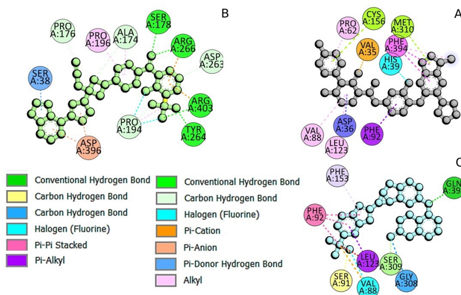
شکل ۱- برهمکنش آنزیم UGT1A1 با A) مرستینیب B) ایتاسیتینیب C) لیفرافنیب. ساختار لیگاندها در وسط هر تصویر و اسیدآمینه های آنزیم در اطراف آن نشان داده شده است. برهمکنش ها با نرم افزار دیسکاواری استودیو بررسی و تصویر آن ذخیره شد.
