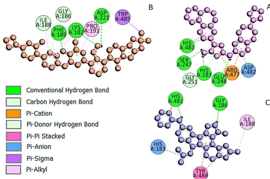
شکل ۳- برهمکنش آنزیم UGT2B7 با A) بمستینیب B) فنبریتینیب C) CEP-11981. ساختار لیگاندها در وسط هر تصویر و اسید آمینه‌های آنزیم در اطراف آن نشان داده شده است. تصاویر به وسیله نرم افزار دیسکاویری استودیو تهیه شدند.
