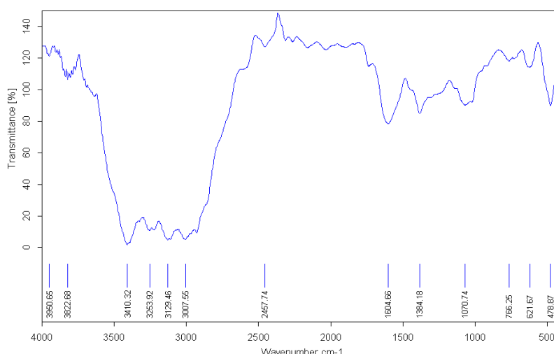
شکل ۳- نتیجه آنالیز با دستگاه FT-IR، دمای 25^\circ\text{C} و pH اسیدی ۴
