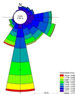
شکل ۵- گلباد هفته اول تا چهارم نمونه برداری (بالا سمت چپ)، گلباد ماه پنجم، هفته پنجم تا هفتم نمونه برداری (بالا سمت راست)، گلباد دو ماه ژوئیه و آگوست. Figure 5. Windrose of the first to fourth week of sampling (left), Windrose of the fifth month, fifth to seventh week of sampling (middle) and Windrose in July and August (right).
