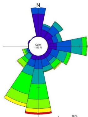
شکل ۵- گلباد هفته اول تا چهارم نمونه برداری (بالا سمت چپ)، گلباد ماه پنجم، هفته پنجم تا هفتم نمونه برداری (بالا سمت راست)، گلباد دو ماه ژوئیه و آگوست. Figure 5. Windrose of the first to fourth week of sampling (left), Windrose of the fifth month, fifth to seventh week of sampling (middle) and Windrose in July and August (right).
