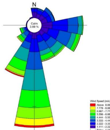
شکل ۵- گلباد هفته اول تا چهارم نمونه برداری (بالا سمت چپ)، گلباد ماه پنجم، هفته پنجم تا هفتم نمونه برداری (بالا سمت راست)، گلباد دو ماه ژوئیه و آگوست. Figure 5. Windrose of the first to fourth week of sampling (left), Windrose of the fifth month, fifth to seventh week of sampling (middle) and Windrose in July and August (right).
