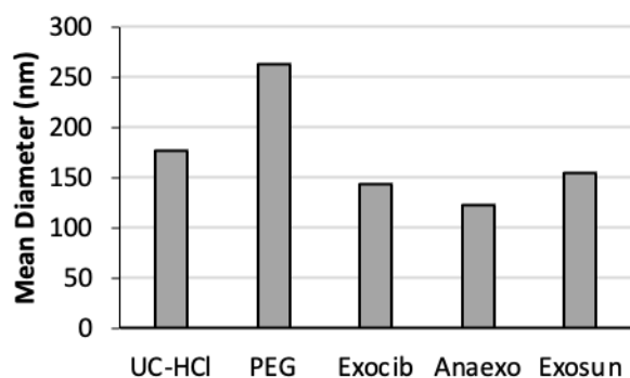
شکل ۲- نمودار مقایسه میانگین قطر ذرات (Mean Size) در روش های مختلف جداسازی اگزوزوم. نمودارها به ترتیب از چپ به راست مربوط به روش های UC-HCl، PEG، Exocib، Anaexo و Exosun می شوند.
