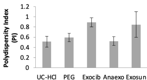
شکل ۳- نمودار مقایسه PI در روش های مختلف جداسازی اگزوزوم. این شاخص نمایانگر میزان هموژن بودن سایز ذرات نمونه پس از جداسازی است. نمودارها مربوط به روش های (به ترتیب از سمت چپ) UC-HCl، PEG، Exocib، Anaexo و Exosun می شوند.
