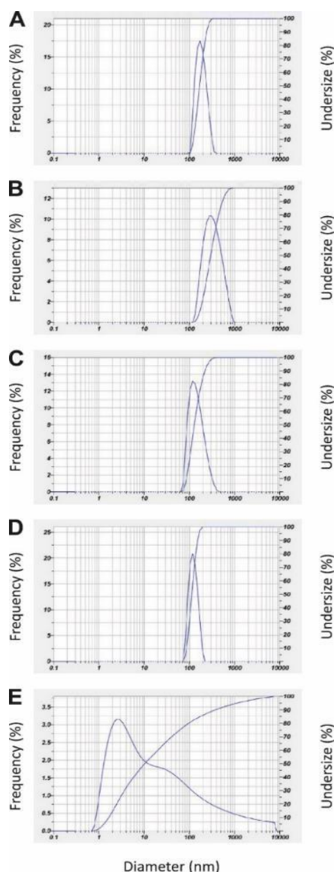
شکل ۱- بررسی اگزوزوم های جداسازی شده توسط روش پراکندگی دینامیکی نور (DLS). سایز و درصد فراوانی ذرات جداسازی شده توسط روش های (A) UC-HCl، (B) PEG، (C) Exocib، (D) Anaexo، (E) Exosun قابل مشاهده است.
