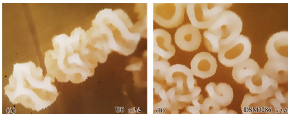
شکل ۱- مقایسه کلنی‌های مخمر Yarrowia lipolytica طبیعی DSM3286 با سویه جهش‌یافته U6. دو سویه بر روی یک پلئیت در شرایط یکسان رشد یافته‌اند. A . سویه جهش‌یافته و B . سویه طبیعی را نشان می‌دهد.
