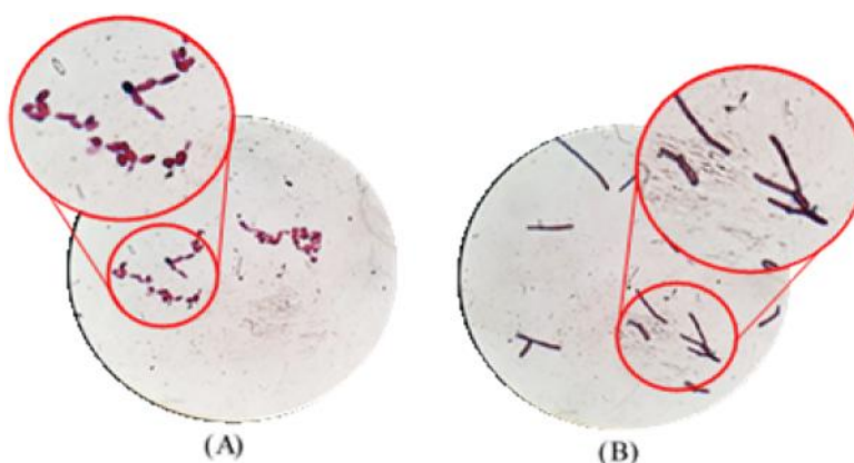
شکل ۲- تصاویر میکروسکوپی از لام مخمر Yarrowia lipolytica (عدسی ۱۰۰×). سلول‌ها به مدت ۱۸ ساعت در محیط YPD مایع رشد کرده‌اند (رنگ آمیزی شده با سافرانین). A. سویه جهش‌یافته U6 در حالت مخمری رشد کرده و B. سویه طبیعی DSM3286 در حالت هیفی رشد کرده است.
