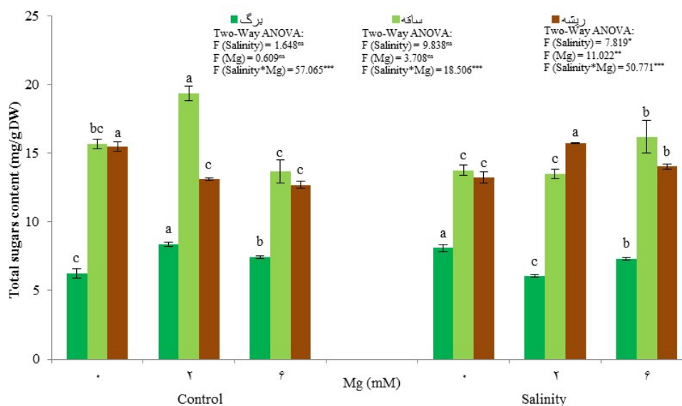
شکل ۳- تاثیر شوری و منیزیم بر محتوای قند کل اسفندک (۴ تکرار \pm SE). حروف یکسان بیانگر عدم اختلاف معنی‌دار در سطح P \leq 0.05 است. *, **, و *** به ترتیب بیانگر معنی‌داری در سطح احتمال ۵، ۱، ۰/۱ درصد و بی‌معنی هستند.
