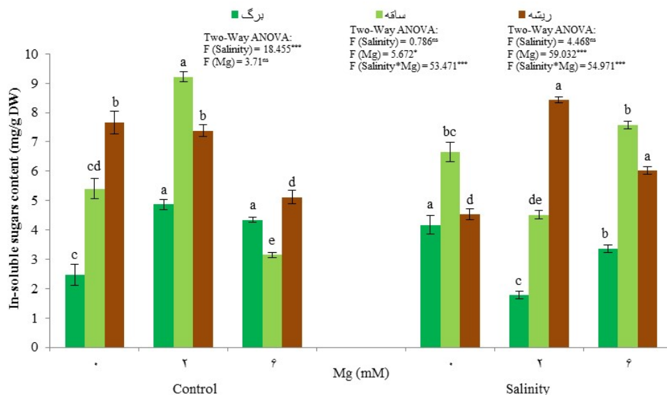
شکل ۲- تاثیر شوری و منیزیم بر محتوای قند نامحلول اسفندک (۴ تکرار \pm SE). حروف یکسان بیانگر عدم اختلاف معنی‌دار در سطح P \leq 0.05 است. *, **, و *** به ترتیب بیانگر معنی‌داری در سطح احتمال ۵، ۱، ۰/۱ درصد و بی‌معنی هستند.
