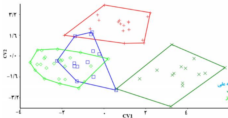
شکل ۵- نمودار تجزیه همبستگی کانونی (CVA)، شکل بدن در جمعیت‌های مورد مطالعه ماهی شیر Schizothorax pelzami . Fig. 5. Canonical variate analysis (CVA) plot of the body shape of the studied Schizothorax pelzami populations.
