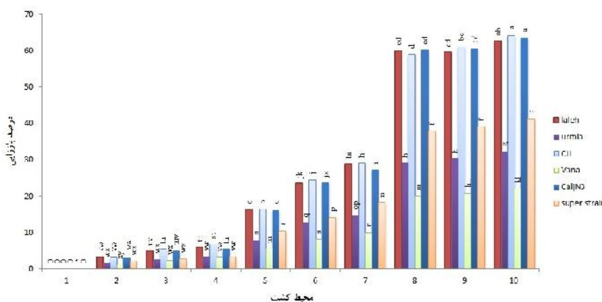
شکل ۱- مقایسه میانگین محیط کشت x رقم. Fig. 1. Comparison of average scores of Media x varieties.
