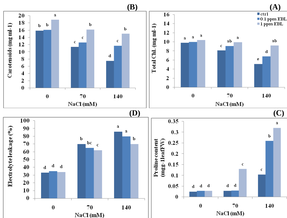
شکل ۲- گیاهان ۳۰ روزه گوجه‌فرنگی که بذرشان با ۲۴-ای‌بی‌براسینولید پرایم شده و تحت تنش شوری رویانده شده‌اند. A: محتوای کلروفیل کل؛ B: غلظت کاروتنوئیدها؛ C: محتوای پرولین آزاد؛ D: نشت الکترولیتی غشاء. میانگین‌های (از سه تکرار) دارای حروف یکسان در سطح ۵ درصد اختلاف معنی‌دار ندارند. Fig. 2. 30-day-old Lycopersicon esculentum plants whose seeds were primed with 24-epibrassinolide and grown under salt stress. A: Total chlorophyll content; B: Carotenoids concentration; C: Free proline concentration; D: Electrolyte leakage. Means (three replicates) with the same letter are not significantly different at p < 0.05 .
