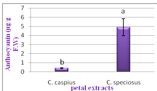
شکل ۴- میزان آنتوسیانین در گلبرگ دو گونه مختلف زعفران. نتایج به صورت میانگین \pm انحراف معیار ارائه شده است ( P \leq 0.05 ).
