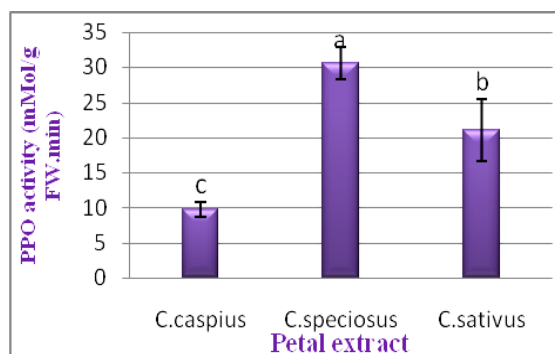
شکل ۷- فعالیت آنزیم PPO در گلبرگ سه گونه مختلف زعفران. نتایج به صورت میانگین \pm انحراف معیار ارائه شده است ( P \geq 0.05 ).
