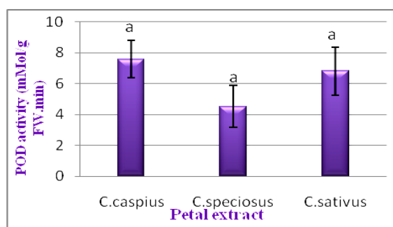
شکل ۶- فعالیت آنزیم POD در گلبرگ سه گونه مختلف زعفران. نتایج به صورت میانگین \pm انحراف معیار ارائه شده است ( P \geq 0.05 ).
