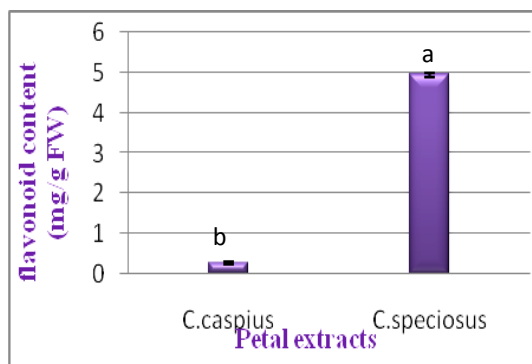
شکل ۵- میزان فلاونوئید در گلبرگ دو گونه مختلف زعفران در طول موج ۳۳۰. نتایج به صورت میانگین \pm انحراف معیار ارائه شده است ( P \leq 0.05 ).
