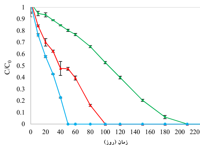
شکل ۱- تخریب PCA در دماهای مختلف (محلول در متانول، نگهداری شده در تاریکی) ۲۵ دمای (■)، ۳۵ دمای (▲)، ۴۵ دمای (●) درجه سانتی‌گراد. Fig. 1. PCA destruction at various temperatures (PCA was kept in methanol in a dark bottle) 25°C (■), 35°C (▲), 45°C (●).
