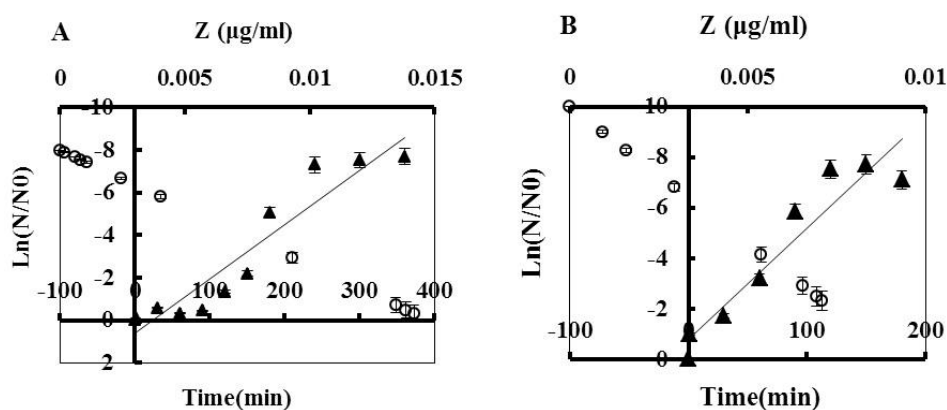
شکل ۳- تغییرات سینتیک مرگ باکتری اشرشیاکلی و مقدار ضریب حساسیت آن. A. غلظت یک برابر مقدار MIC. B. غلظت دو برابر مقدار MIC (▲ Iron oxide NP-kinetics, Iron oxide NP-Z value). اکسید آهن-سینتیک، نانو ذره اکسید آهن - مقدار (Z).
