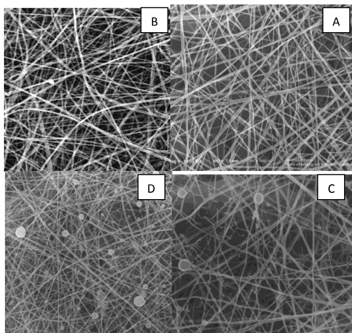
شکل ۱- تصویر میکروسکوپ الکترونی روبشی (SEM) نانوالیاف پلیمری الکتروریسی شده. A: Chit/PEO 90:10، B: Chit/PEO/Li 1%، C: Chit/PEO/Li 2%، D: Chit/PEO/Li 3%.
