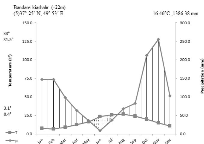
شکل ۲- نمودار منحنی آمبروتیک ایستگاه هواشناسی بندر کياشهر (۲۰۰۷-۲۰۱۲).
