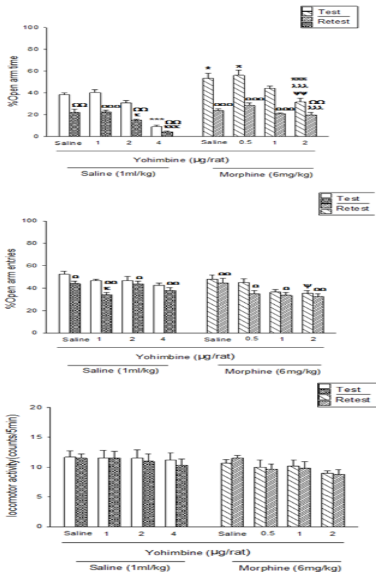
شکل ۳- تأثیر تزریق یوهیمبین درون BLA، به تنهایی یا همراه با مورفین بر رفتارهای شبه اضطرابی و به خاطرآوری حافظه.
