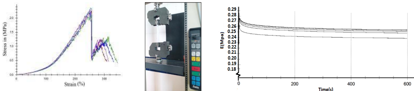
شکل ۱. نتایج آزمون مکانیکی پارچه A03، (الف) آزمون کشش، (ب) تصویر دستگاه زوئیک (ج) آزمون رهاسازی تنش
