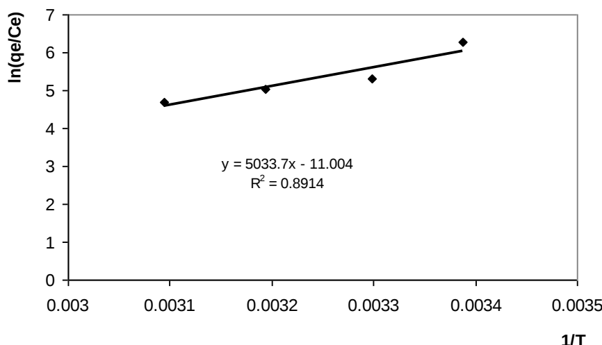
شکل ۵. منحنی تغییرات \ln \left( \frac{q_e}{C_e} \right) بر حسب 1/T برای به‌دست آوردن پارامترهای ترمودینامیکی (غلظت اولیه جذب‌شونده: 0.1 \text{ M} ، دما: 295\text{--}323 \text{ K} ، مقدار جاذب: 3/5 \text{ g} ) جدول ۲. پارامترهای ترمودینامیکی جذب فرمیک اسید روی کربن رنگبر
