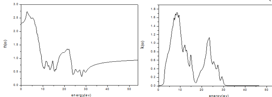
شکل ۷: نمودار سمت راست مربوط به ضریب خاموشی، نمودار سمت چپ مربوط به ضریب شکست ترکیب SrS در ساختار NaCl
