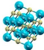
شکل ۱. ب) ساختار CsCl سولفید استرانسیوم
