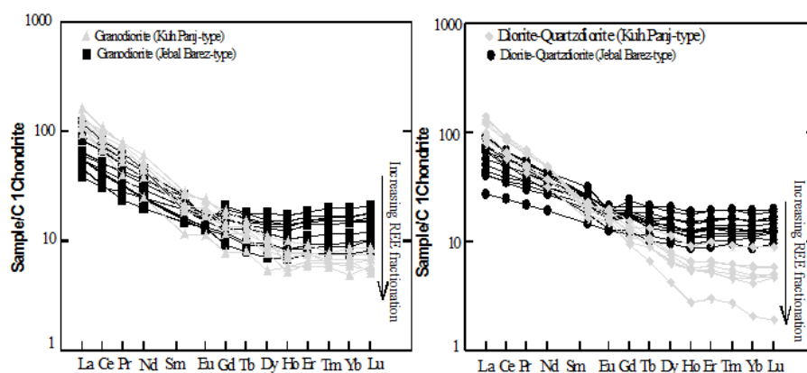
شکل ۷. مقایسه الگوی تغییرات فراوانی عناصر خاکی نادر در توده‌های نفوذی تیپ جبال بارز و تیپ کوه پنج که نسبت به کاندريت C1 به‌هنجار شده‌اند. غنی‌شدگی کمتر گرانیتوئیدهای کوه پنج از عناصر خاکی نادر متوسط و سنگین نسبت به گرانیتوئیدهای جبال بارز به‌وضوح با قرار گرفتن روندهای مربوط به عناصر مذکور در آن‌ها در زیر روندهای مربوط به گرانیتوئیدهای جبال بارز آشکار است
