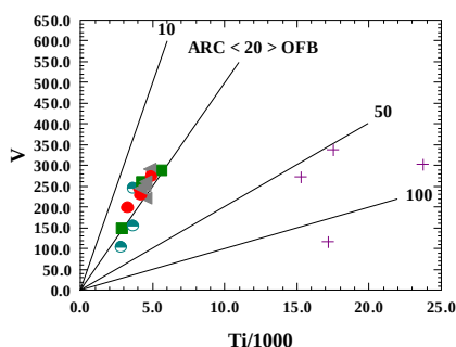
شکل ۵. نمودار متمایز کننده بازالت‌ها براساس Ti-V [۱۸] 10 < Ti/v < 20 = تولیت‌های جزایر قوسی 20 < Ti/v < 50 = بازالت‌های طغیانی قاره‌ای و مورب 50 < Ti/v < 100 = بازالت‌های جزائر اقیانوسی و بازالت‌های آکالن Ti/v = 20 = بازالت‌های کالکوالکالن
