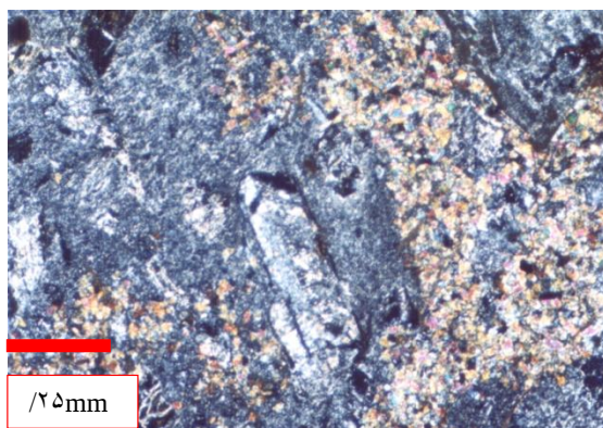
شکل ۸. دگرسانی بازالت آندزیتی در پهنه سیرسیتی (XPL* 4)
