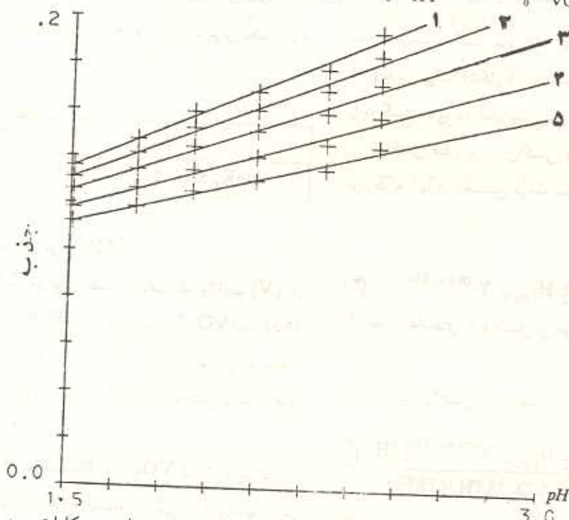
شکل ۲ - نمایش تغییرات جذب \text{VO}_2^+ بر حسب pH در قدرت یونی یک مول بر لیتر پراکلات سدیم در 30^\circ\text{C} و در طول موجهای (۱) ۲۶۰، (۲) ۲۶۵، (۳) ۲۷۰، (۴) ۲۷۵، (۵) ۲۸۰ نانومتر. C_{\text{VO}_2} = 1/1000 \times 10^{-4} \text{M}
