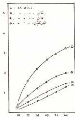
شکل ۹- مقایسه تاثیر الکل های متانل، اتانل و اتیلن گلیکول روی حذف آهن از ایلمنیت احیا شده در غلظت ۰/۵ مولار HCl
