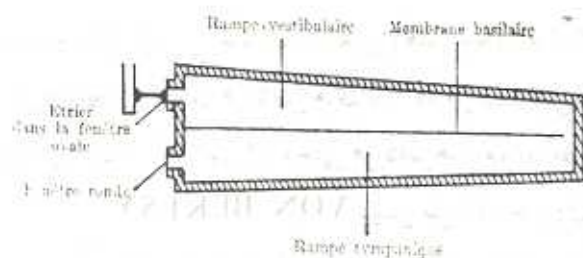
شکل ۲ حلزون نمونه Von Bekesy
