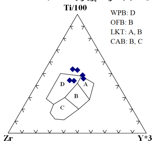
شکل ۸. نمودار متمایز کننده Ti-Zr-Y برای بازالت‌ها [۹]. LKT : تولیت‌هایی با پتاسیم کم، CAB : بازالت‌های کالک آلکالن، OFB : بازالت‌های کف اقیانوسی و WPB : بازالت‌های درون قاره‌ای.
