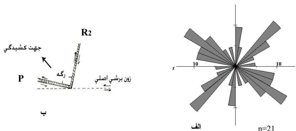
شکل ۱۰. (الف) نمودار گل سرخی راستای رگه‌های منظم، (ب) هم‌خوانی راستای رگه‌ها و شکستگی‌های ریدل (R2) و P در شکل ۱۱ الف مشاهده می‌شود که محور تعدادی از بودین‌ها عمود بر محور چین‌ها هستند در حالی‌که در اصل باید این دو موازی هم باشند. راستای محور این بودین‌ها شمال باختری است و لذا فشارش شمال خاوری- جنوب
