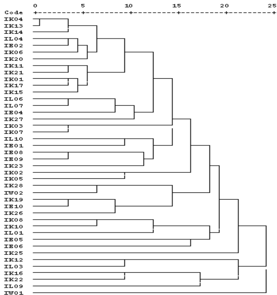
شکل ۵. دندروگرام حاصل از تجزیه خوشه‌ای بر اساس محصولات RAPD
