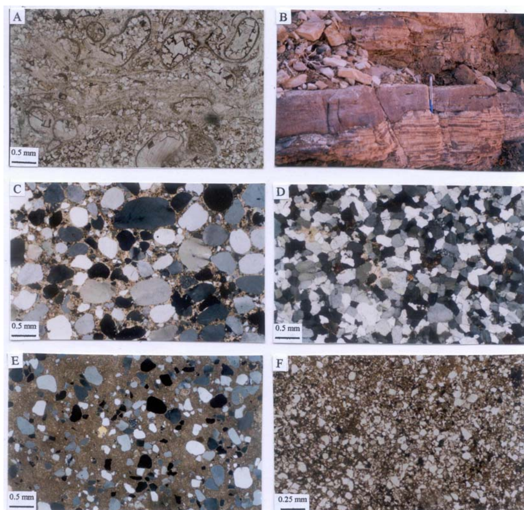
شکل ۵- A- تصویر دیگری از گریستون بیوکلاستی (به رخساره طوفانی کریناته). آلوک‌های تشکیل دهنده Claraia و Spirobis هستند. نمونه کوارتزهای آواری و بلورهای اتومورف دولومیت نیز دیده می‌شوند (نمونه از برش گذار گچال، نور طبیعی) B- نمونه‌ای از رخنمون رخساره طوفانی کریناته که دارای سطح زیرین ناگهانی و فرسایشی است (برش گذار گچال) C- کوارتز آرنیت (رخساره N) در این تصویر، کوارتزهای بایمدال در زمینه‌ای از سیمان کلسیتی دیده می‌شوند (نمونه از برش گذار گچال، نور پلاریزه) D- تصویر دیگری از کوارتز آرنیت (رخساره N) کوارتزها به فرم بایمدال بوده و تلفیقی از سیمان‌های سیلیسی، کلسیتی و دولومیتی در زمینه مشاهده می‌شود (نمونه از برش گذار گچال، نور پلاریزه) E- کوارتز وک (زیر رخساره O1) کوارتزها به فرم بایمدال هستند (نمونه از اسلام آباد، نور پلاریزه) F- لیتیک گریوک (زیر رخساره P1) در این تصویر، لیتوکلاست‌ها از خرده سنگ‌های آهکی بوده‌اند که توسط بلورهای اتومورف دولومیت، جانشین شده‌اند (نمونه از برش گذار گچال، نور پلاریزه)
