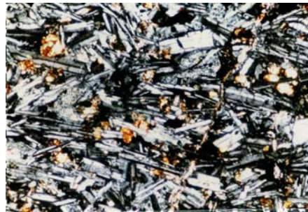
شکل ۱۳- بازالت تا حدی دگرسان شده با بافت پیلوتاکیستی (بزرگ‌نمایی 25\times ، xpl).
