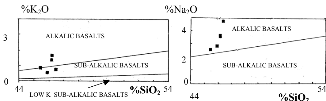
شکل ۵- طبقه‌بندی بازالت‌های آلوکالیک و ساب آلوکالیک (نقل از میدل ماست ۱۹۷۵، اقتباس از ویلسون ۱۹۹۷)
