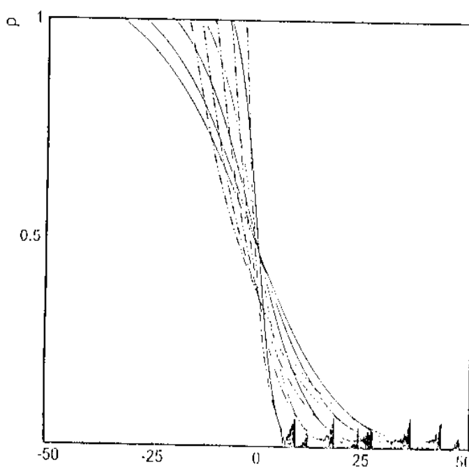
شکل ۵: تحول زمانی چگالی پلاسما به ازاء A = 3 ، \Omega = 0.8 و \gamma = 1 . نمودار با خط ممند بدون ذرات محبوس نمودار نقطه چین با ذرات محبوس
