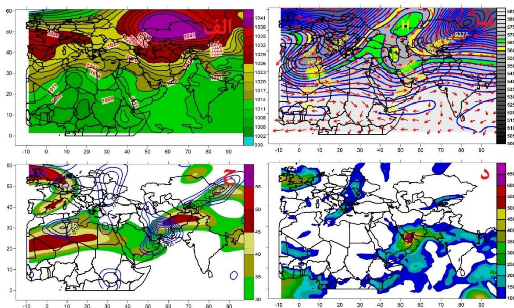
شکل ۴. الف) فشار سطح دریا به پاسکال (ب) ارتفاع ژئوپتانسیل تراز ۵۰۰ هکتوپاسکال به متر و جهت جریان باد تراز ۵۰۰ هکتوپاسکال (ج) امگا تراز ۵۰۰ به پاسکال و رودباد تراز ۲۵۰ هکتوپاسکال به متر بر ثانیه (د) رودخانه جوی کیلوگرم متر بر ثانیه
