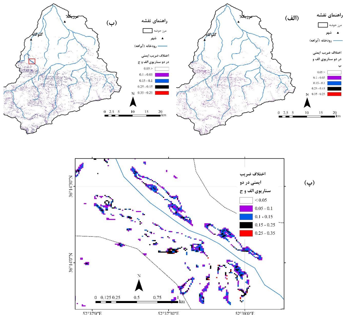
شکل ۱۵- اختلاف ضریب ایمنی حداقل در حوضه آبخیز مورد مطالعه برای شرایط مختلف: (الف) بعد از گذشت ۶ ساعت از شروع بارش؛ (ب) بعد از گذشت ۱۸ ساعت از شروع بارش و (پ) نمایش بخشی از نقشه با بزرگنمایی بیشتر (کادر قرمز رنگ در شکل ب) بررسی نقشه‌های ارائه شده در شکل ۱۵ نیز نشان می‌دهد که افت ضریب ایمنی پایداری بعد از وقوع بارندگی‌ها باز هم در بخش‌هایی از زون ۶ که در بخش‌های مرتفع حوضه قرار دارند، بیشتر از نقاط دیگر حوضه رخ داده است. این موضوع نیز با مشاهدات صحرایی همخوانی خوبی نشان می‌دهد، به طوری که بعد از وقوع بارندگی‌های طولانی مدت، ناپایداری‌های دامنه‌ای از نوع لغزش‌های کم عمق و جریان گلی-واریزه‌ای در بخش‌های مرتفع حوضه بیشتر از سایر نقاط اتفاق می‌افتند. البته لازم به ذکر است که اینگونه زمین لغزش‌ها به دلیل عدم وجود جاده دسترسی مناسب، صعب العبور بودن و غیرمسکونی بودن این بخش‌ها، وسعت و عمق کم و عدم اثرگذاری مستقیم بر سکونتگاه‌ها و جاده‌های روستایی منطقه، کمتر شناسایی شده و معمولاً در بانک‌های اطلاعاتی موجود ثبت نمی‌شوند، اگرچه، به دلیل افزایش پتانسیل فرسایش خاک و تأمین مصالح جریان‌های واریزه‌ای می‌توان به طور نسبی آنها را با اهمیت در نظر گرفت. نکته دیگری که از بررسی این نقشه‌ها قابل استنتاج است، این
