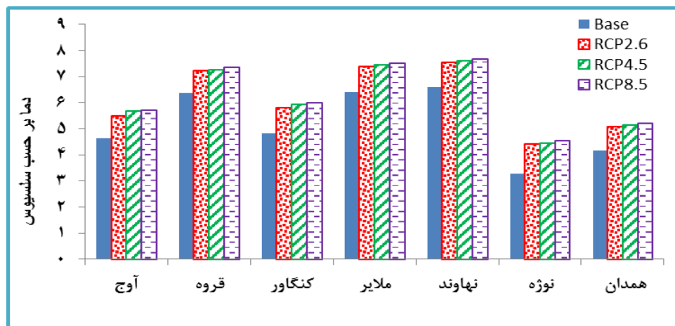
شکل ۶. متوسط بلندمدت دمای کمینه در دوره آینده نسبت به دوره پایه بر اساس سناریوهای مختلف
