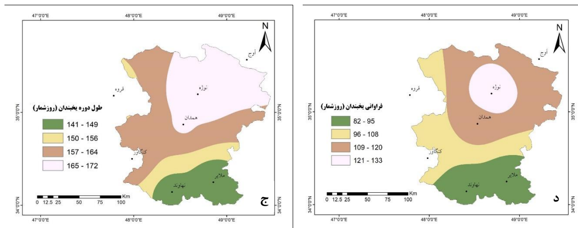
شکل ۳. میانگین تغییرات مکانی فراوانی وقوع و طول دوره یخبندان در منطقه مورد مطالعه بر حسب روز در بازه ۱۹۹۰ تا ۲۰۲۰
