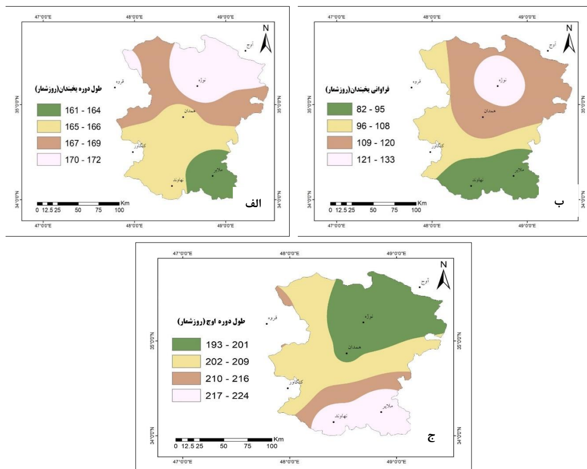
شکل ۴. میانگین طول دوره، فراوانی وقوع و دوره اوج یخبندان در ایستگاه‌های استان در بازه ۱۹۹۰ تا ۲۰۲۰
