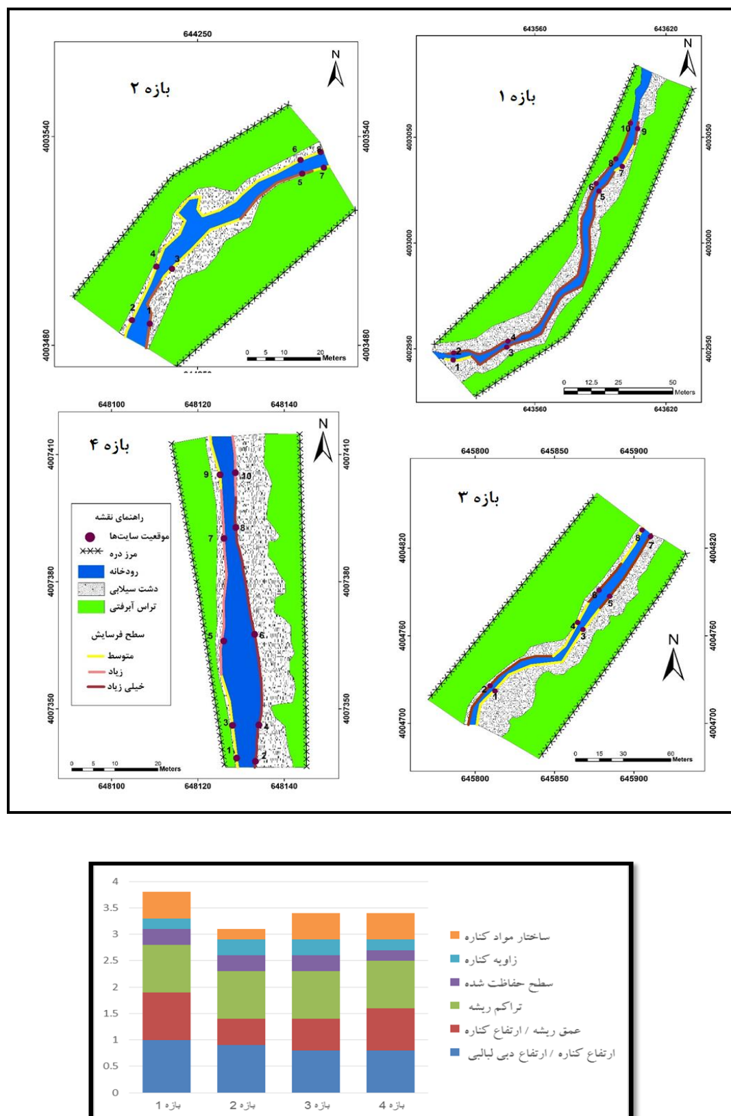
شکل ۵. طبقه‌بندی فرسایش‌پذیری کرانه رود در بازه‌های مورد مطالعه رودخانه سجادرود با روش BEHI
