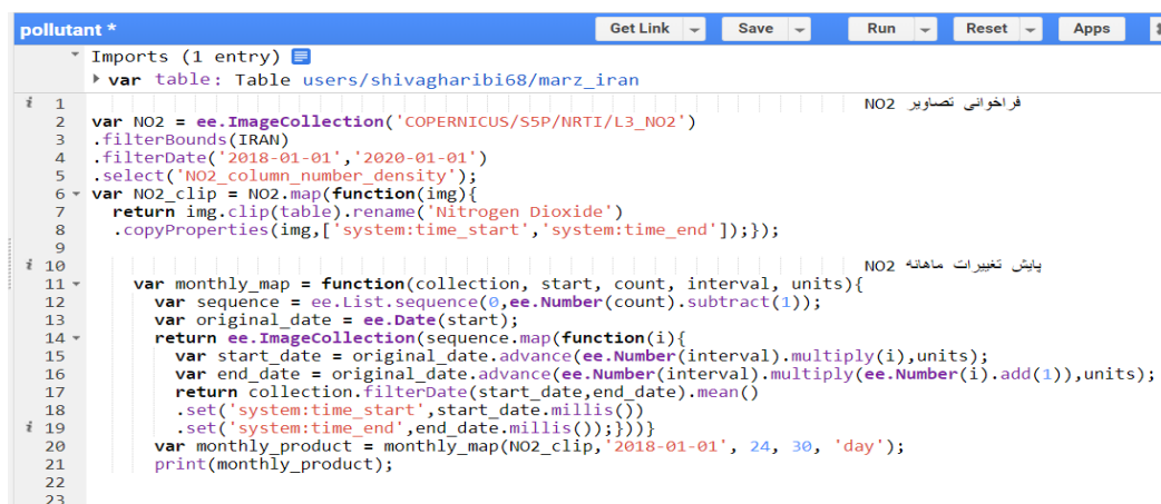
شکل ۲: نمونه Script اجرا شده برای فراخوانی تصاویر سنتینل جهت پایش تغییرات \text{NO}_2
