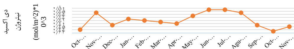
شکل ۴: نمودار تغییرات میانگین ماهانه آلاینده NO ۲ در طول ۲۰۱۸-۲۰۱۹
