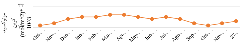
شکل ۳: نمودار تغییرات میانگین ماهانه آلاینده CO در طول ۲۰۱۸-۲۰۱۹
