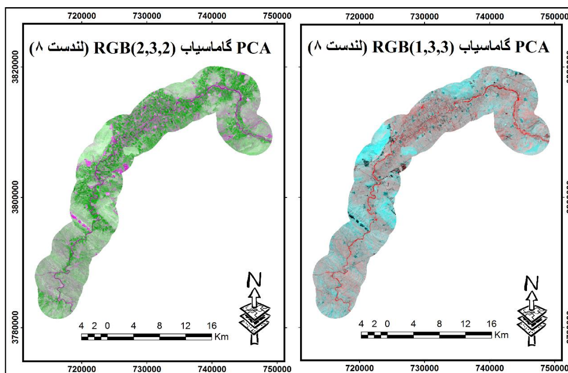
شکل ۴. تحلیل مولفه‌های اصلی بر روی سنجنده OLI
