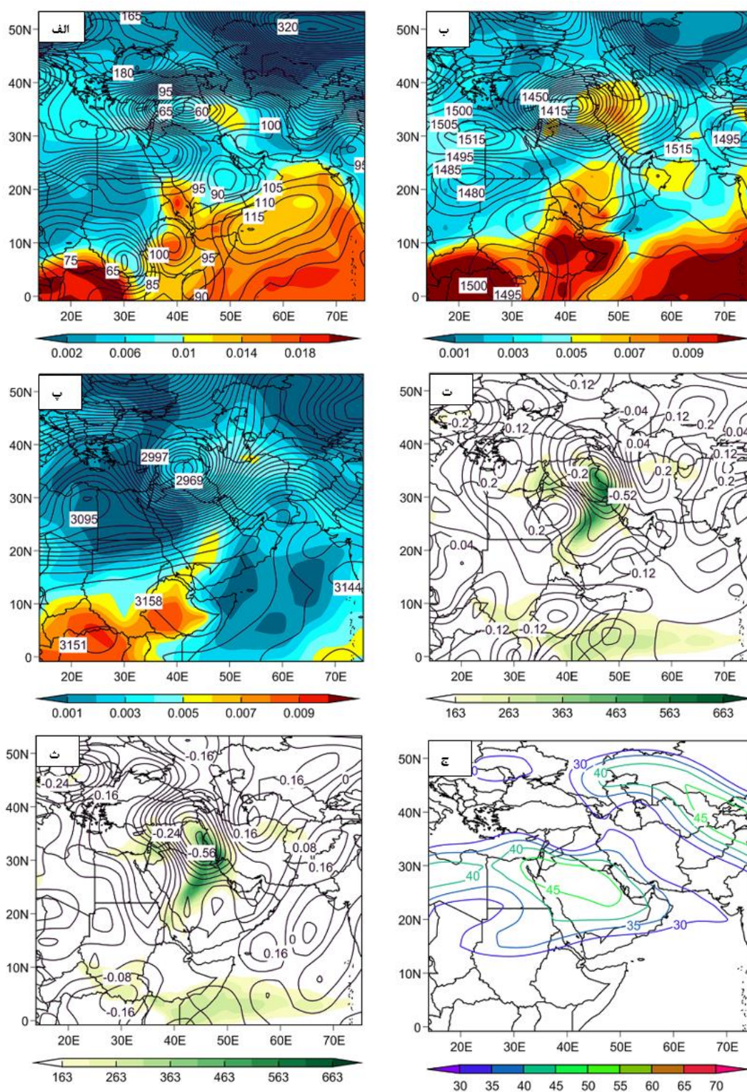
شکل ۱۳. الف) نقشه ترکیبی ژئوپتانسیل متر و نم و یژه به کیلوگرم در کیلوگرم روز ۱۸ فوریه ۲۰۱۸ (تراز ۱۰۰۰، ب) تراز ۸۵۰ و پ) تراز ۷۰۰ هکتوپاسکال، ت) نقشه ترکیبی رودخانه (IVT) در ساعت اوج به همراه امگای تراز ۷۰۰ و ت) تراز ۵۰۰ هکتوپاسکال، ج) نقشه جت تراز ۲۵۰ هکتوپاسکال
