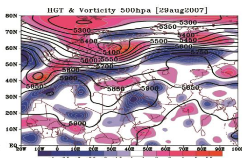
شکل ۸. وضعیت ارتفاع ژئوپتانسیل و تاوایی تراز ۵۰۰ هکتوپاسکال (الگوی اول)
