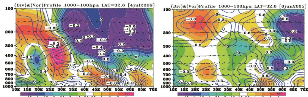
شکل ۱۸. نیمرخ قائم تاوایی و واگرایی برای عرض ۳۲
