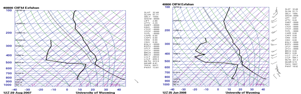
شکل ۲۹. نمودار اسکیتی ایستگاه اصفهان (الگوی دوم)
