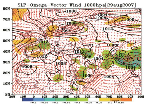
شکل ۱۳. وضعیت فشار، امگا و بردار باد در سطح زمین (الگوی دوم)
