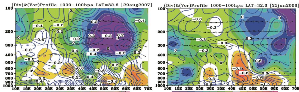
شکل ۱۶. نیمرخ قائم تاوایی و واگرایی برای عرض
