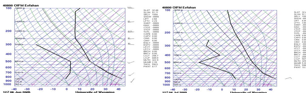
شکل ۳۱. نمودار اسکیتی ایستگاه اصفهان (الگوی چهارم)
