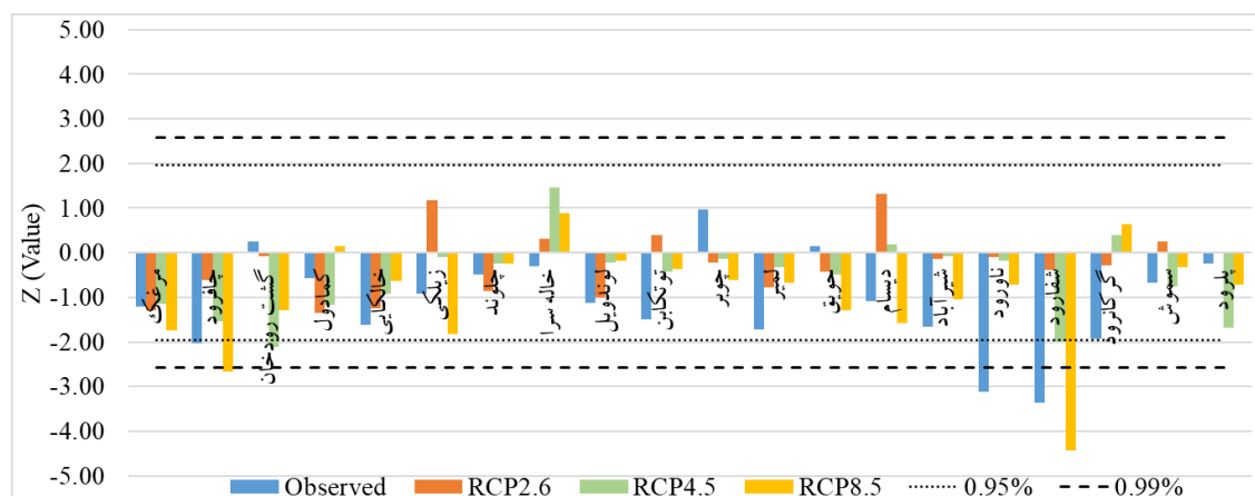
شکل ۵. مقادیر (Z) داده‌های مشاهداتی و مدل شده‌ی دبی جریان رودخانه‌ها با سناریوهای RCP_{2.6} ، RCP_{4.5} و RCP_{8.5}
