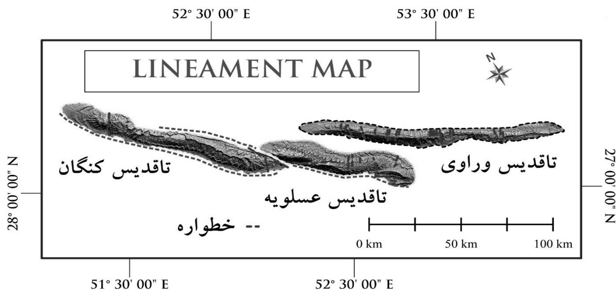
شکل ۴. نقشه خطواره‌های مهم تکتونیکی تاکدیس‌های مورد مطالعه
