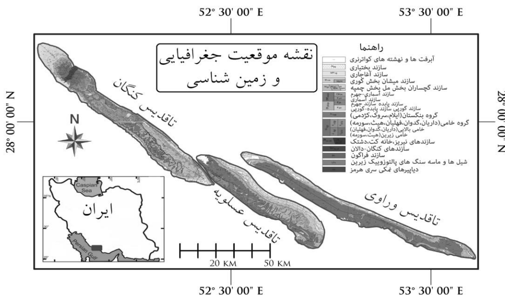
شکل ۲. موقعیت جغرافیایی و زمین شناسی منطقه مورد مطالعه
