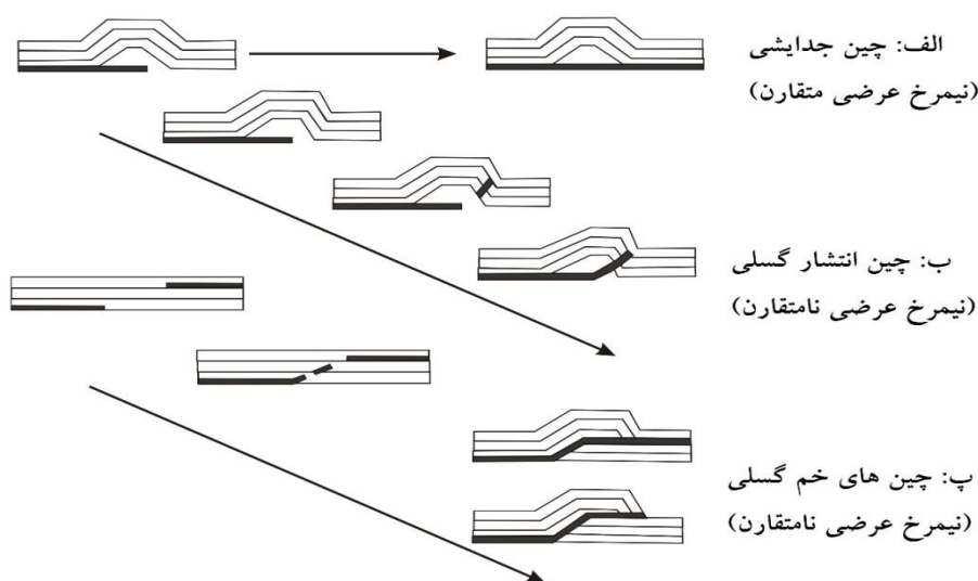
شکل ۱. سازوکار ساده شده ایجاد سه نوع از چین خوردگی‌ها (برگرفته از باربری و همکاران، ۲۰۱۰، ۱۴۰)
