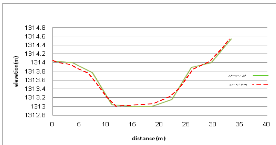
شکل ۸: مقطع عرضی ۵ قبل و از شبیه سازی
