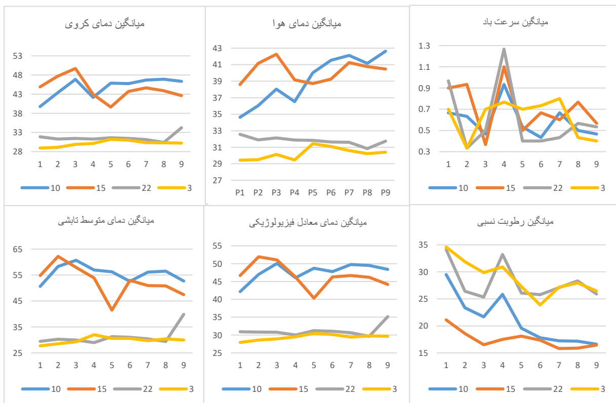
شکل ۵. نتایج میانگین داده های اولیه و ثانویه در ۴ ساعات اندازه گیری ۱۰ صبح، ۳ بعدازظهر، ۱۰ شب و ۳ بامداد.
