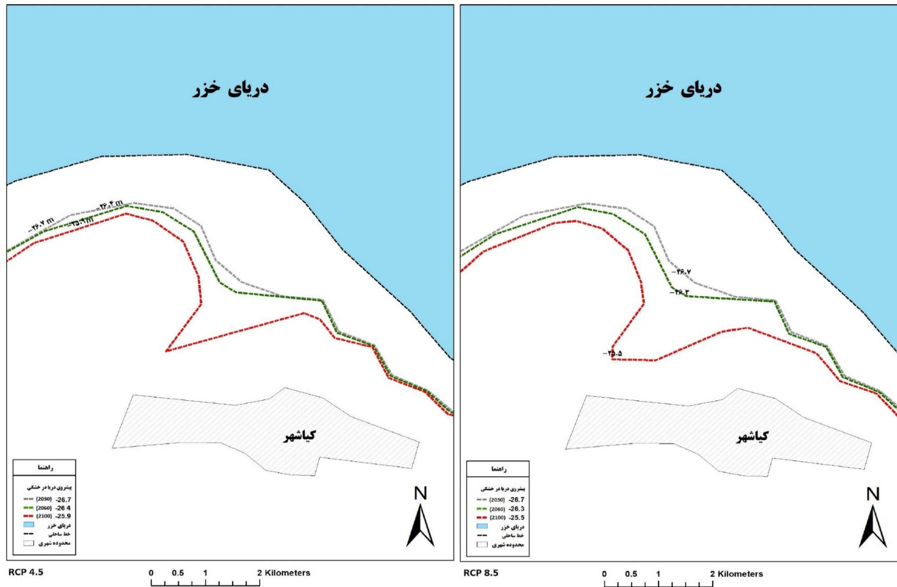
شکل ۱۷: پیش بینی محدوده عقب نشینی خط ساحلی کیاشهر در سناریوی RCP 4.5 و RCP 8.5
