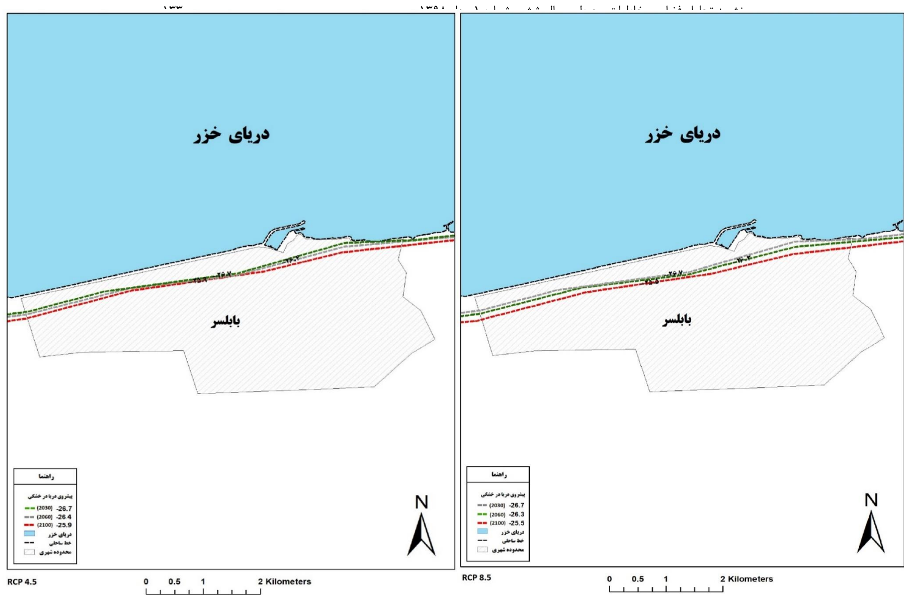
شکل ۱۸: پیش بینی محدوده عقب نشینی خط ساحلی بابلسر در سناریوی RCP 4.5 و RCP 8.5
