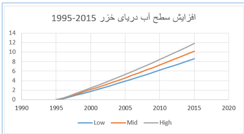
شکل ۱۰: تغییرات سطح دریای خزر ۱۹۹۵-۲۰۱۵
