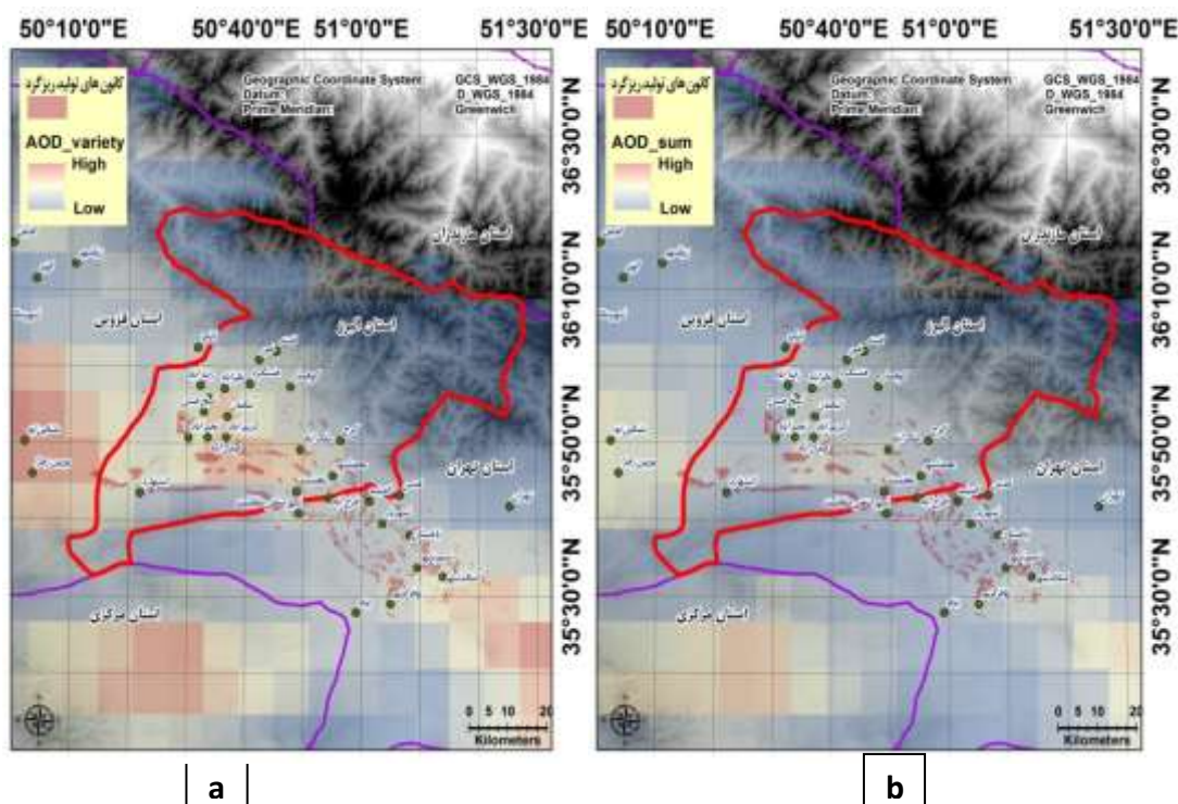
شکل ۶- نقشه ارزیابی صحت کانون‌های تولید ریزگرد به کمک تغییرات آماری عمق اپتیکی هواویز سال ۲۰۱۰ تا ۲۰۱۵
