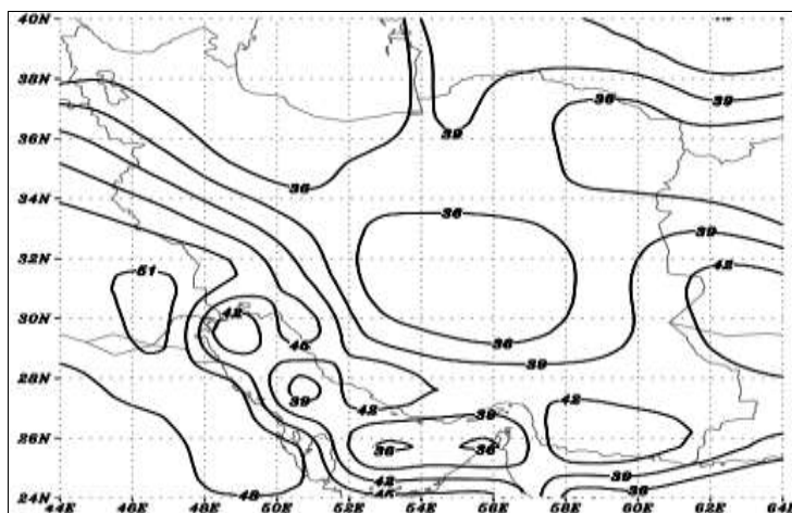
شکل ۹. دمای بیشینه دومتري سطح زمين در گرم ترين روز موج گرمايي ضعيف ۱۱ ژوئيه ۱۹۸۱
