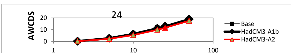
شکل ۱۲: شدت تجمعی خشکسالی به ترتیب از بالا به پایین برای برای تداوم زمانی ۳، ۱۲ و ۲۴ ماهه در دوره مشاهداتی، A1B و A2 و برای دوره برگشت ۲ تا ۵۰ سال برای مناطق مرکزی ایران
