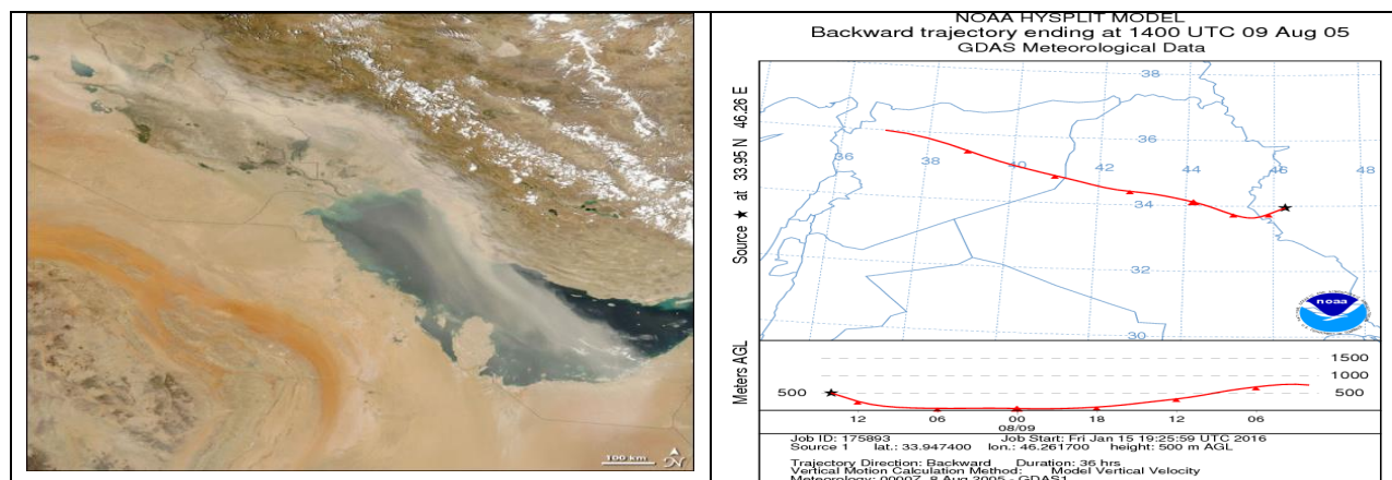
شکل ۴: الف) اجرای مدل HYSPLIT به روش Backward در روز ۱۸ مرداد ۱۳۸۴ (ساعت ۱۴) تصویر مدیس روی ماهواره آکوا در روز ۱۷ مرداد ۱۳۸۴
