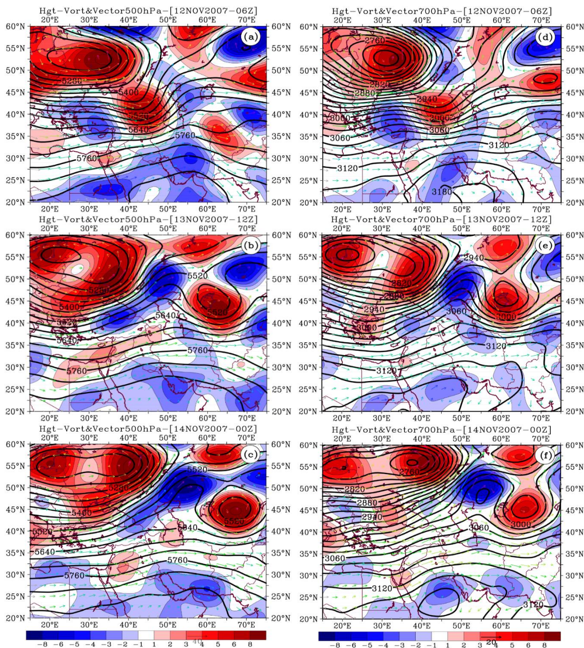
شکل ۳) وضعیت همدیدی در الگوی پرفشار مهاجر برای ساعات مختلف روزهای آلوده. ارتفاع ژئوپتانسیل (کنتورها با حداصل ۲۵ ژئوپتانسیل متر)، تلاوایی نسبی (رنگ ها s^{-1} \times 10^{-4} ) و باد برداری (پیکان های سبز رنگ) در تراز ۵۰۰ (سمت چپ) و تراز ۷۰۰ هکتوپاسکال (سمت راست).
