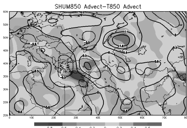
شکل ۱۳: فرارفت رطوبت ویژه (مقادیر رنگی شده بر حسب درجه‌ی سلسیوس بر ثانیه) و فرارفت دما (خطوط هم‌مقدار) در تراز ۸۵۰ هکتوپاسکال برای ساعت ۰۶ دسامبر ۲۰۰۹.
